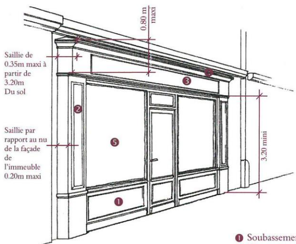
Schéma d'une devanture en applique
