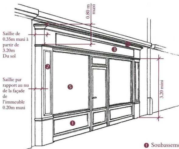
Schéma d'une devanture en applique
