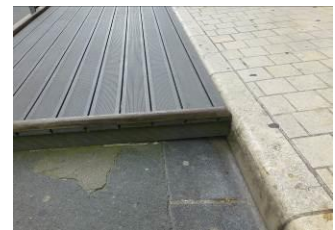
Lorsqu'on doit faire un platelage temporaire de mise à niveau d'un trottoir, celui-ci ne doit pas excéder la hauteur du trottoir ; celui-ci peut aussi être réalisé en tôle d'acier de ton gris.
